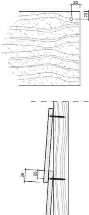
невидимое (основное) крепление
