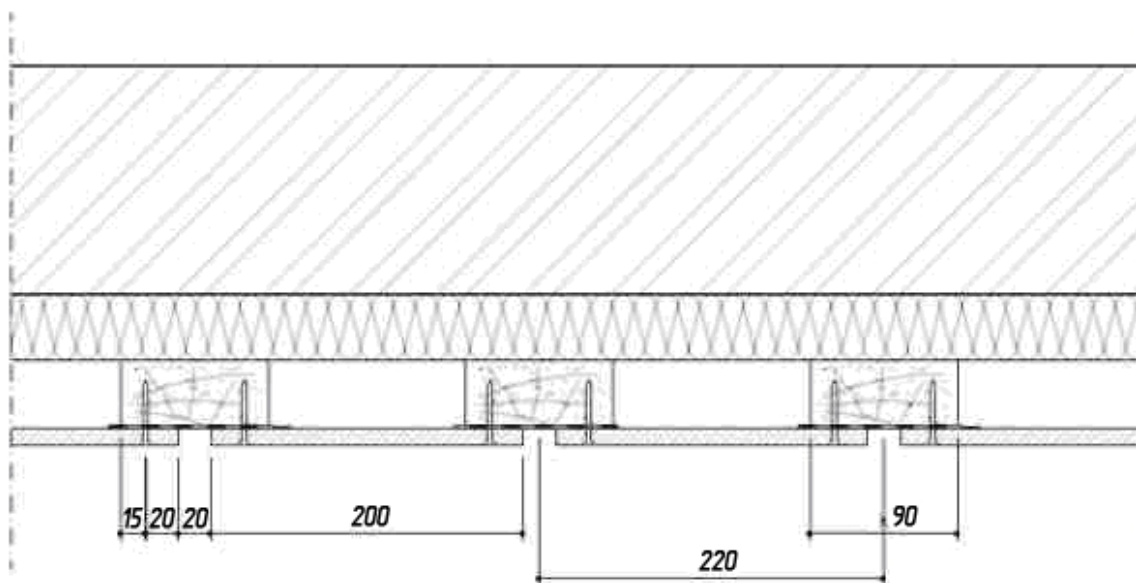
Вертикальное крепление LATONIT - сайдинга с открытым швом (Тип В).
