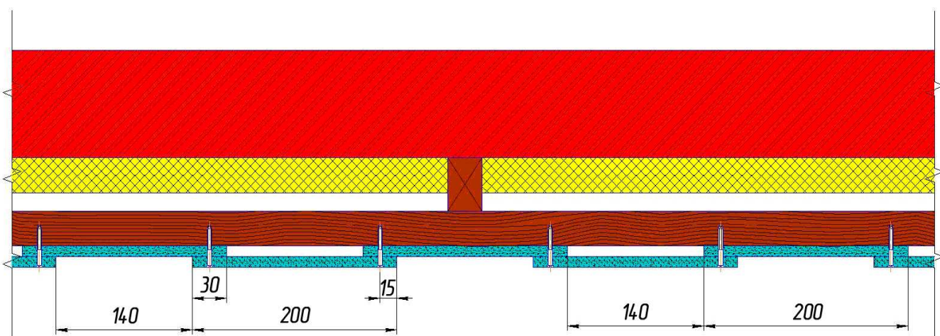
Вертикальное крепление LATONIT - сайдинга с закрытым широким швом (Тип Б)
