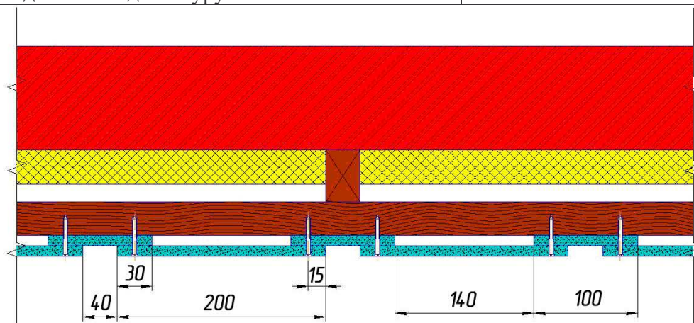
Вертикальное крепление LATONIT - сайдинга с закрытым узким швом (Тип А)
