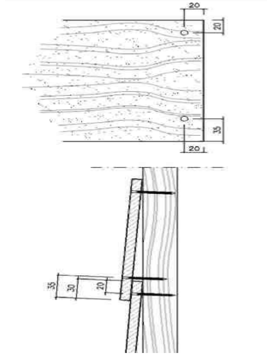
видимое (дополнительное) крепление
